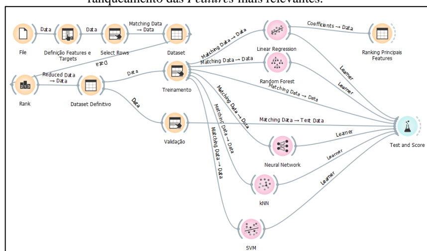
Figura 1 - Esquete desenvolvido no Orange-Canvas para filtro do dataset , aplicação dos algoritmos e ranqueamento das Features mais relevantes.
