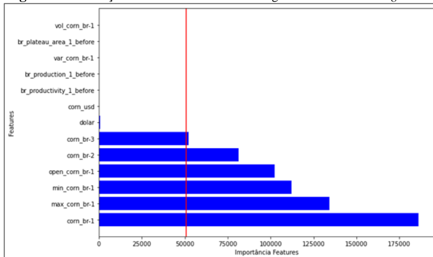
Figura 2 - Pontuação das Features baseado no algoritmo Univariate Regression
